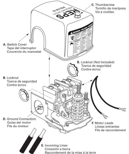
Figure 2. Parts Drawing Figura 2. Dibujo de las piezas Figure 2. Dessin de pièces
